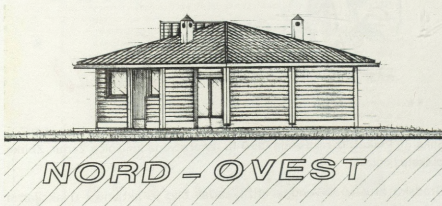
Slika 80: Preslik iz dijela nacrtu dječjega vrtića koji je realiziran donacijom Udruge volontera „Solidariet Vigolana“. (Gradsko društvo Crvenog križa Zadar)
